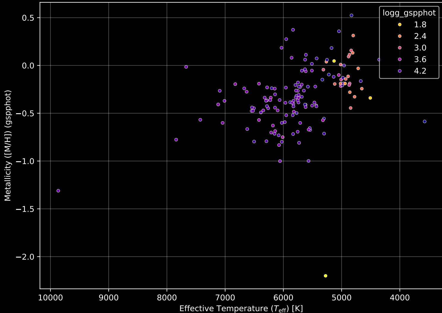
GALAH DR4 Field: [7240] Stellar Population Parameters (n= 145)
