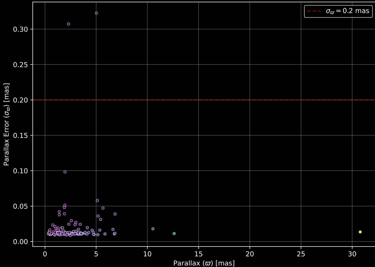
GALAH DR4 Field: [7240] Parallax Quality (n= 145)
